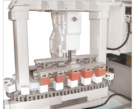
Bild 1: Logica Macro 5 Farben mit Ovaalem Taktband Mod. Speedway für Druck auf Papierklötzen
